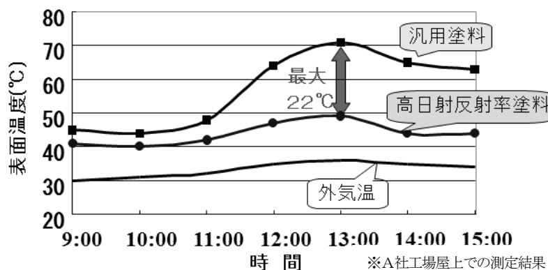
高日射反射率塗料と汎用塗料の表面温度変化
