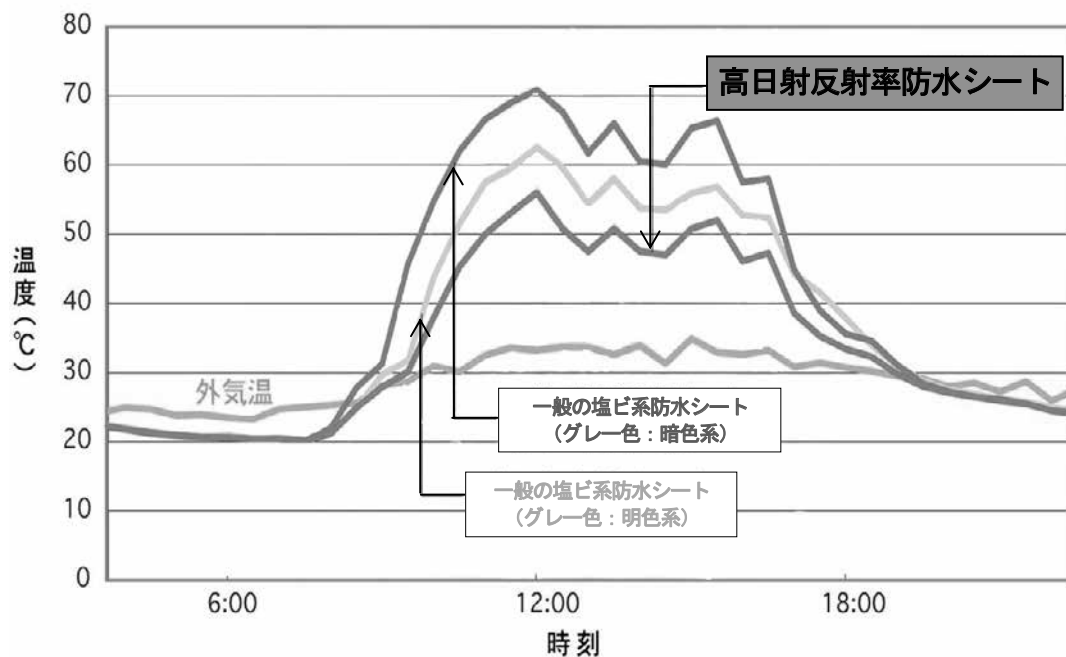
高日射反射率防水シートと一般シートの表面温度変化の例
