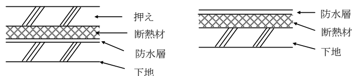
押え工法
